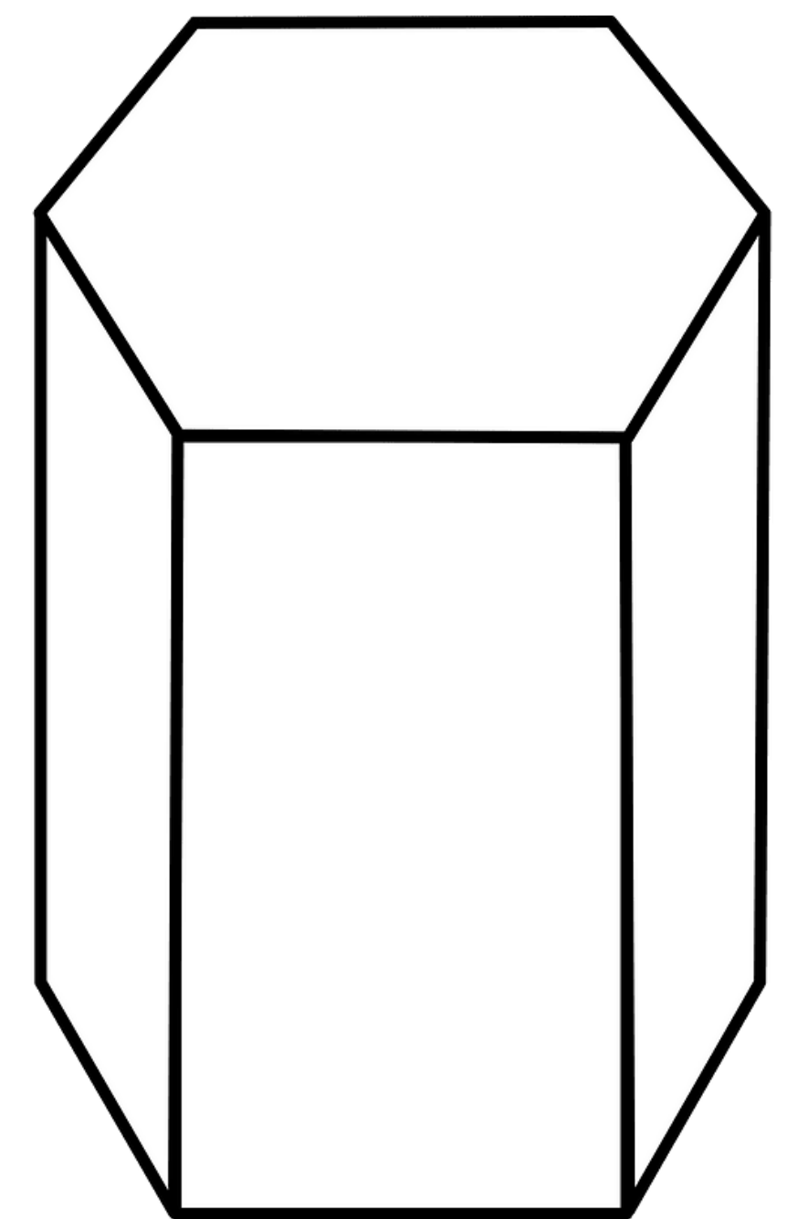
graniastosłup prawidłowy sześciokątny
