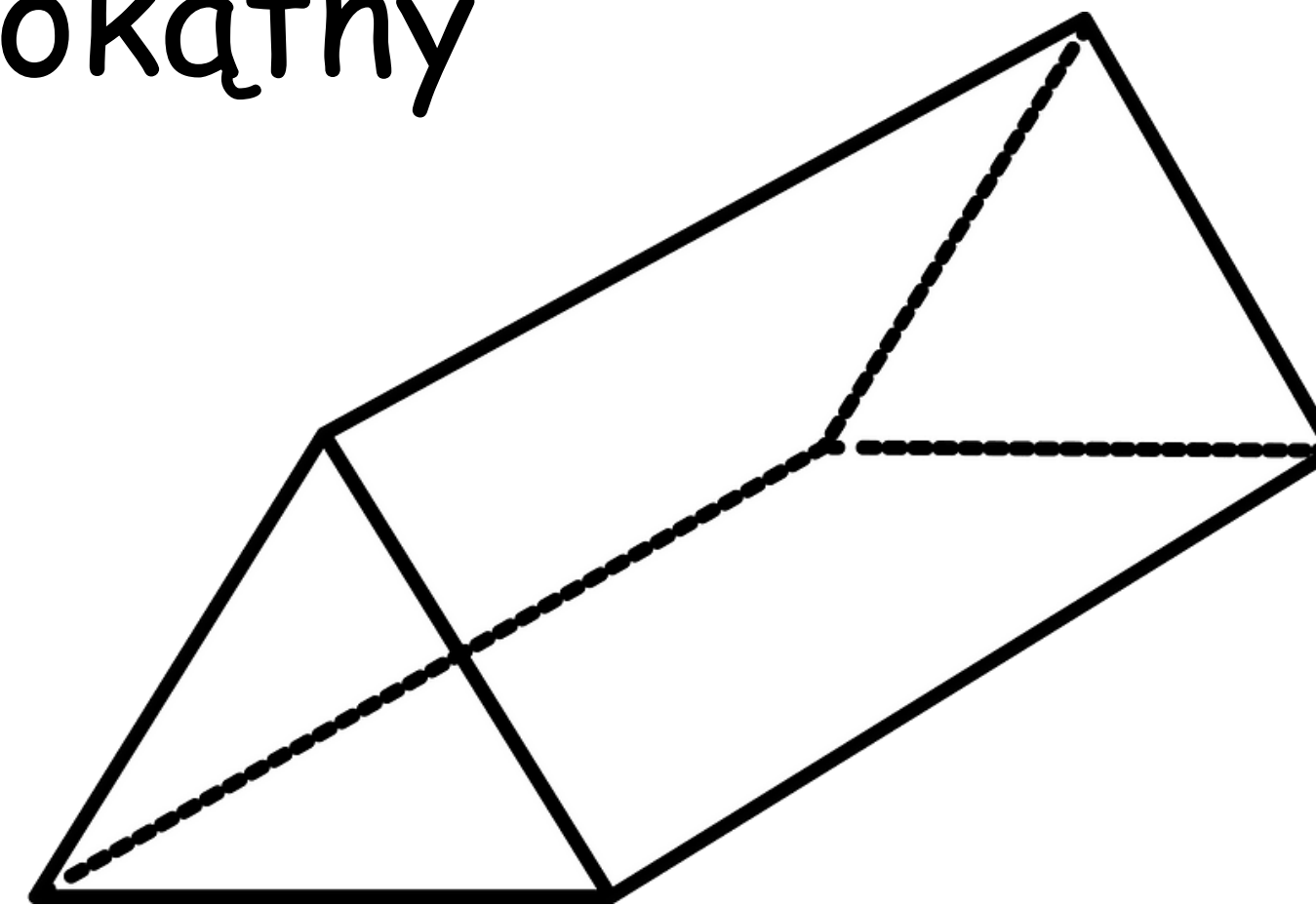
graniastosłup prawidłowy trójkątny
