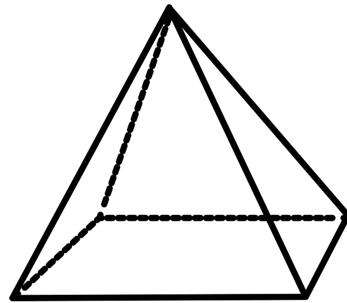
ostrosłup prawidłowy czworokątny
