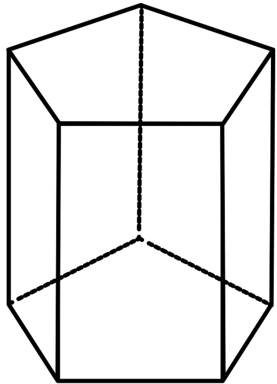
graniastosłup prawidłowy pięciokątny
